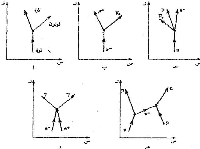
الشكل (4-1) الخطوط العالمية لأحداث مختلفة في دنيا الجسيمات (أ) انبعاث فوتون من ذرة (ب) انحلال بايون (ج) انحلال بيتا السالب (د) فناء بوزترون - إلكترون (هـ) عملية تبادل بايون.
