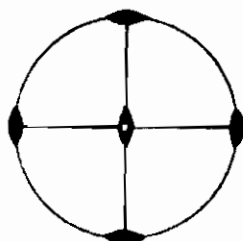
Orthorhombic
