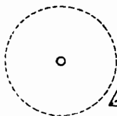
Triclinic
